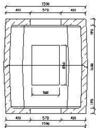
Przekrój poprzeczny
