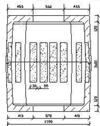
Przekrój poprzeczny
