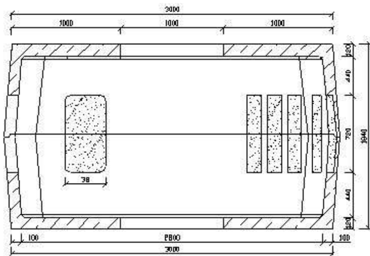
Przekrój poziomy
